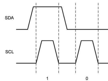
그림 1. START, STOP 조건 사이의 데이터 비트 송수신 타이밍
