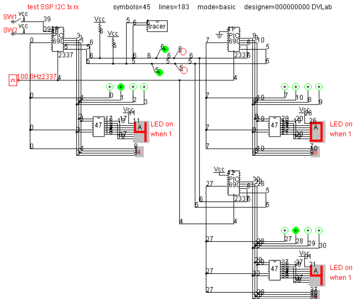
그림 3. I2C 모듈 기능 검증을 위한 예제 회로도
