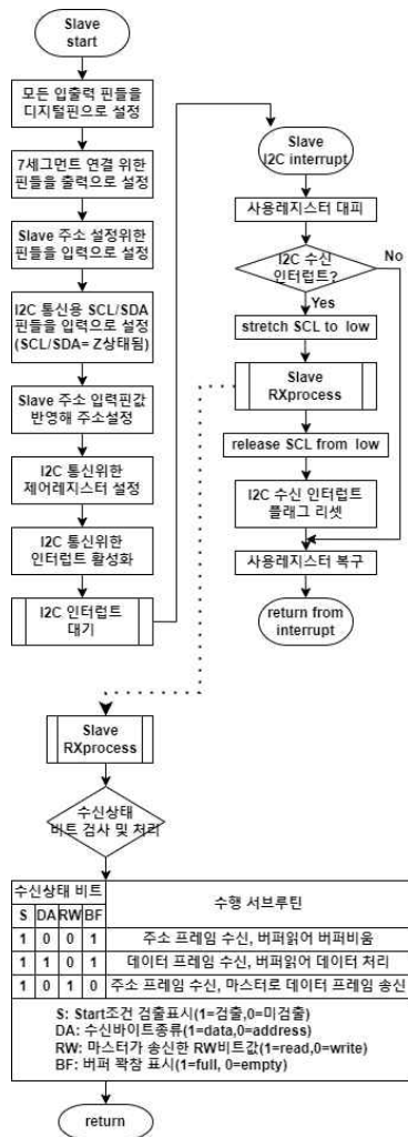
그림 5. 슬레이브 프로그램 흐름도 Fig. 5. Slave program flowchart
