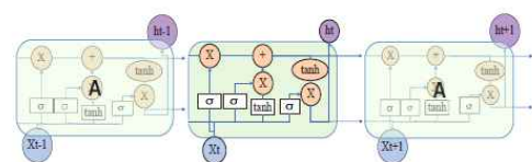
그림 1. LSTM 네트워크 구조 개략도[2]
