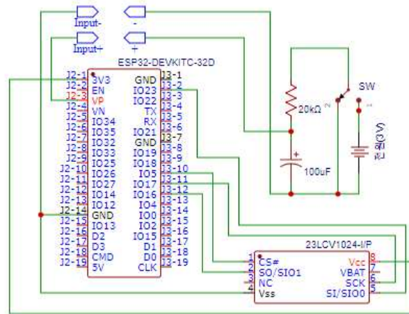
그림 3. 측정장치 회로도
