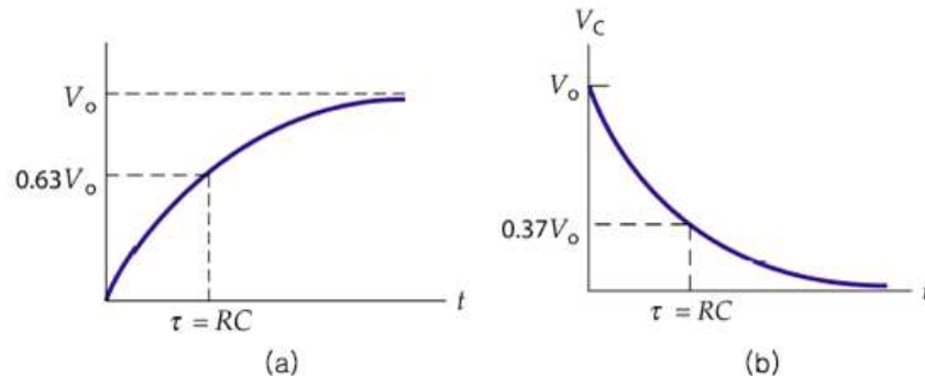
그림 1. RC 회로에서 충전(a)과 방전(b)할 때 시간에 따른 축전기 양단 전압의 변화
