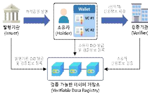
그림 1. SSI 모델 기반 분산신원증명 기술 흐름도 Fig 1. SSI model-based DID Flowchart
