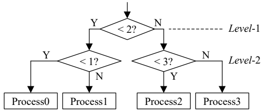
그림 2. 트리 구조 if문
