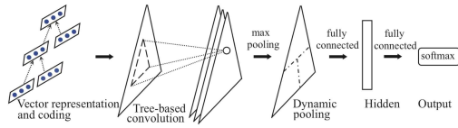
그림 4. TBCNN의 신경망 구성 Fig 4. Organization of TBCNN
