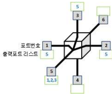
그림 5. 3차원 스위치 동작 예(1:3 연결) Fig. 5. 3D switch operation(1:3 connection)
