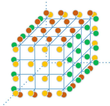
그림 1. 4x4x4 3차원 스위치 연결 구조 Fig. 1. 4x4x4 3-dimensional switch connection architecture
