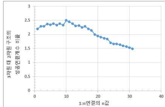
그림 7. 3차원 대 2차원 구조의 성공연결개수 비율 Fig. 7. Ratio of the number of successful connection in 3D/2D architecture
