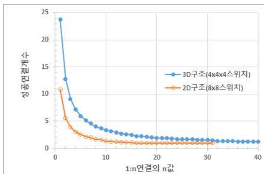
그림 6. 성공연결개수 비교 Fig. 6. Comparison of the number of successful connection
