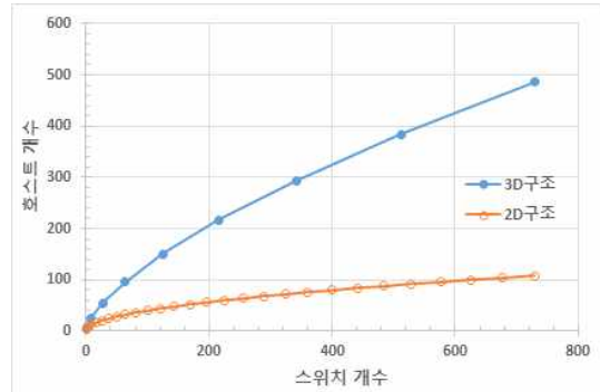
그림 3. 스위치 구조별 수용가능 호스트 수 Fig. 3. Number of affordable hosts in 3D/2D architecture
