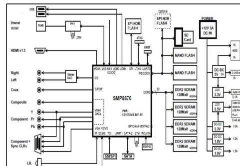
그림 2. IPTV 개발보드의 부품 구성도
