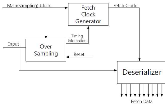
그림 6. 오버샘플링 회로 블록도
