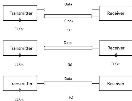
그림 2. 시리얼링크의 클록킹 방식 (a)포워드드 클록킹 (b)임베디드 클록킹 (c)임베디드 클록킹(레퍼런스 없는) Fig. 2. Clocking schemes of the serial link (a)forwarded clocking (b) embedded clocking and (c) embedded clocking(reference-less)
