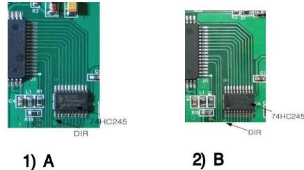
그림 3. 동일 데이터 전달방향 사용예
