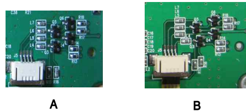
그림 4. 수동소자의 동일 배치 사용예
