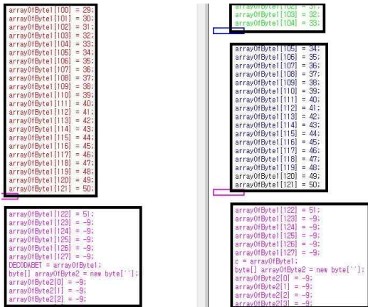
그림 3. 기법 1의 변수 선언부 패턴 매칭
