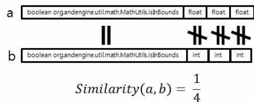
그림 2. 메서드간의 유사도 측정
