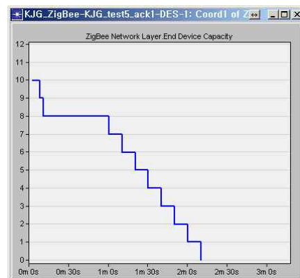
그림 4. Association Flood 공격에 따른 코디네이터의 허용 단말노드 수 변화
