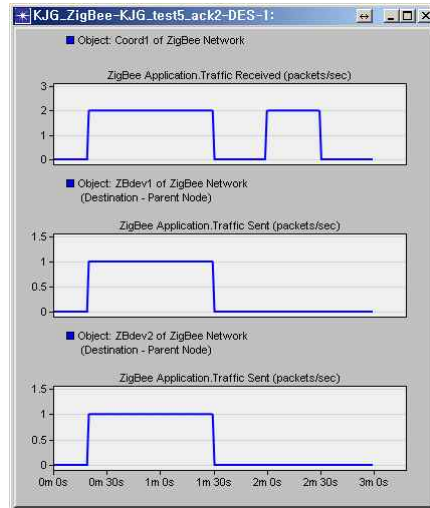
그림 6. Replay 공격에 따른 코디네이터 수신 데이터 및 단말노드 송신 데이터 변화
